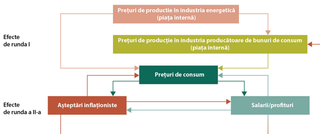
Grafic C. Canale de transmisie a variației prețurilor de producție din industria energetică în variația prețurilor de consum
