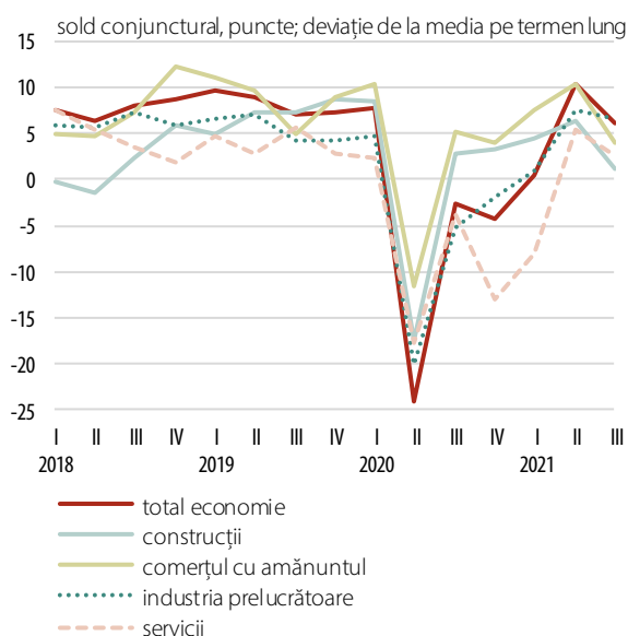
Grafic 2.13. Așteptările operatorilor economici privind numărul de salariați în următoarele 3 luni*
