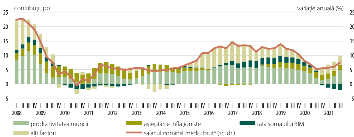
Grafic 2.14. Contribuția factorilor determinanți la dinamica salariului mediu brut pe economie 26
