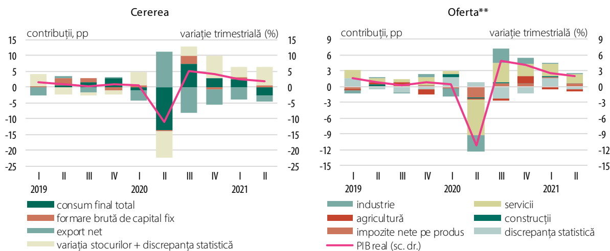
Grafic 2.1. Contribuții la creșterea economică*
