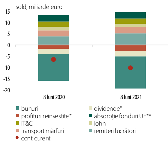
Grafic 2.9. Contul curent și principalele componente
