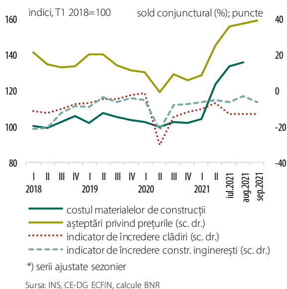
Grafic 2.6. Indicii ale perspectivei în construcții*
