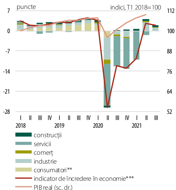
Grafic 2.2. PIB și sentimentul economic*
