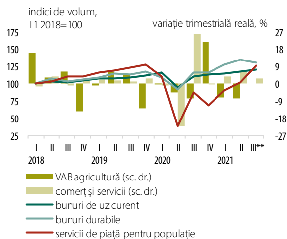
Grafic 2.3. Achizițiile comerciale și sectorul agricol*
