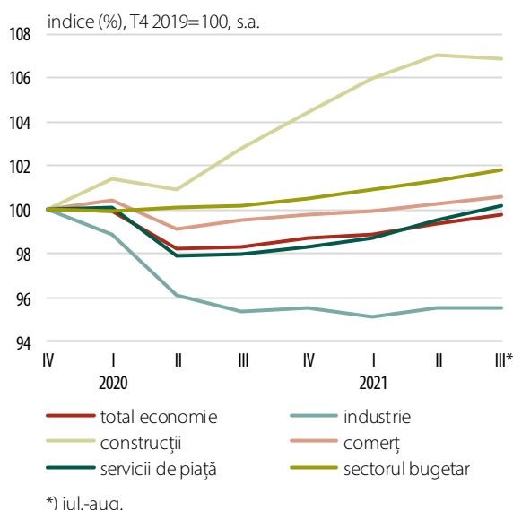
Grafic 2.12. Efectivul salariaților din economie
