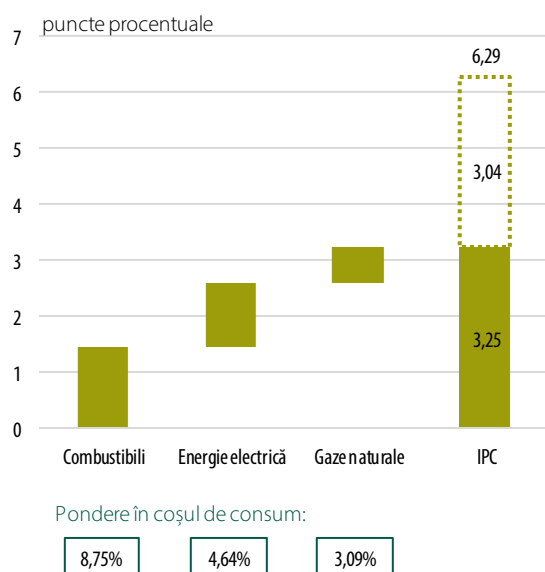
Grafic 1.3. Contribuția energiei la inflația IPC
