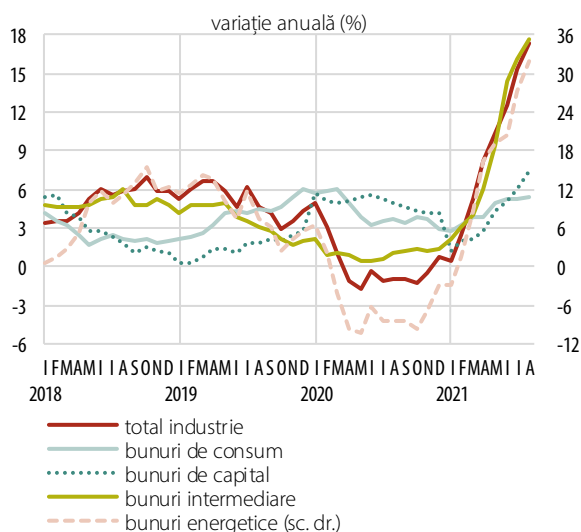
Grafic 2.16. Prețurile producției industriale pentru piața internă
