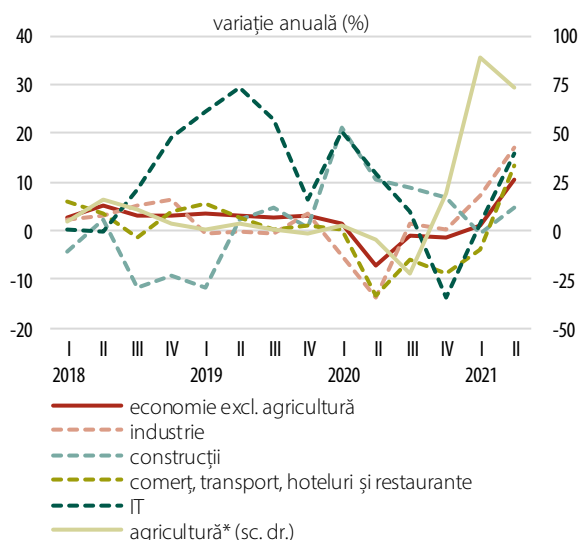
Grafic 2.10. Productivitatea muncii în economie
